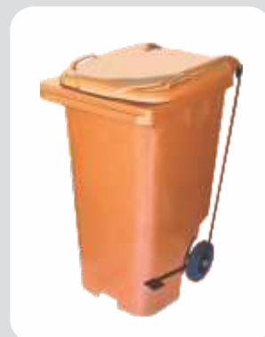
CONTENTOR PLÁSTICO COM RODAS 200mm E PEDAL LATERAL 1060x570x720mm Capacidade: 240L
